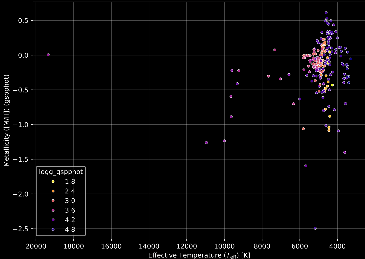
APOGEE DR17 Field: [100-18_btx] Stellar Population Parameters (n= 259)
